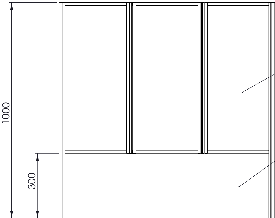
SEZIONE B-B
