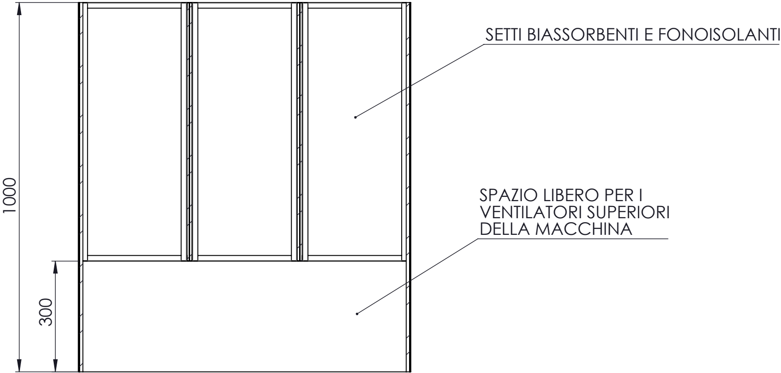
SEZIONE A-A
